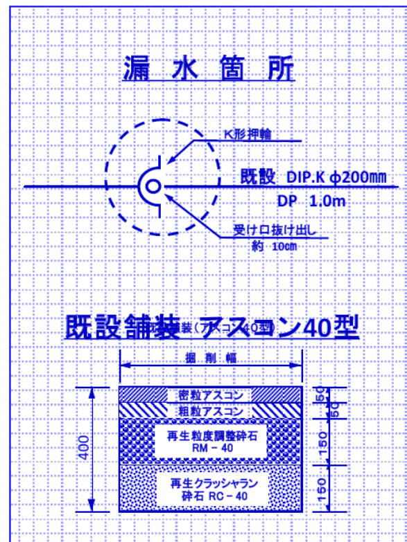
配管図 (施工前)
