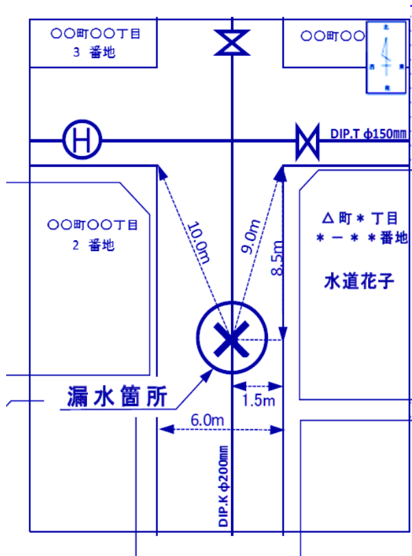
現場見取り図
